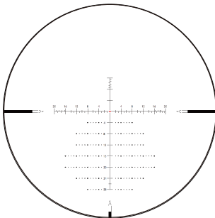
VSE-4 MOA Reticle Pattern
