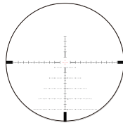
VSE-5 MOA Reticle Pattern
